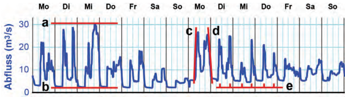
Abbildung 3.1: Schwallbeeinflusste Abflussganglinie am Beispiel der Vispa bei Visp während zwei Wochen anfangs März 2012. Rot hervorgehoben sind die Parameter zur hydrologischen Beschreibung der Schwallereignisse: a: Q_{max} , b: Q_{min} , c: \Delta Q_{Schwall} , d: \Delta cm/s_{Sunk} , e: Häufigkeit der Schwallereignisse (verändert nach BAFU Hydrologie 2012).
