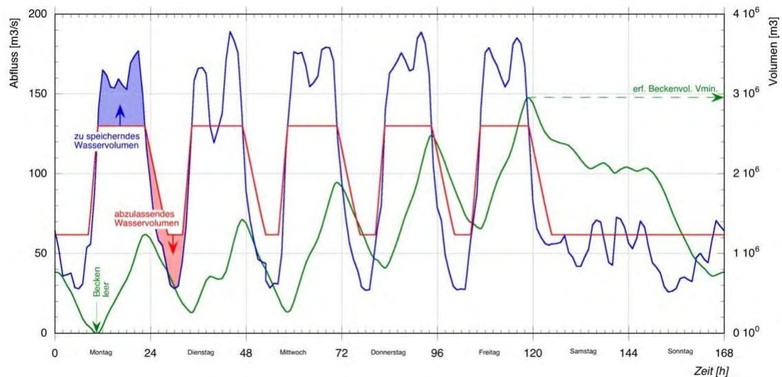
Abbildung 4.1: Beispiel einer gedämpften Abflussganglinie (aus Baumann et al. 2012). In diesem Beispiel könnte das Schwall/Sunk-Verhältnis während einer ganzen Woche durch ein Beruhigungsbecken mit einem Volumen von ca. 3 Mio m 3 von ca. 7:1 auf etwas über 2.1:1 reduziert werden. Gleichzeitig könnten weitere Schwall/Sunk-Parameter wie Abflussextrême und Abflussänderungsraten deutlich verbessert werden (rote Linie).
