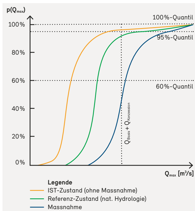
Abb. E3 Summenhäufigkeit, dargestellt am Beispiel des Schwallabflusses Q_{max} .
