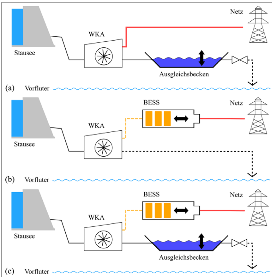
Bild 2: Integration von Schwall-Sunk-Sanierungsmaßnahmen: (a) nur Ausgleichsbecken, (b) nur BESS und (c) hybrides Becken-BESS (WKA: Wasserkraftanlage, BESS: Batterie-Energiespeichersystem).
